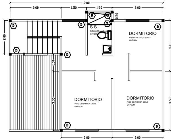
SEGUNDO NIVEL
