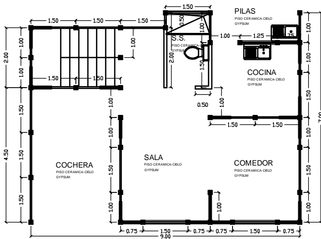
PRIMER NIVEL
