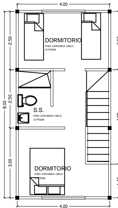
SEGUNDO NIVEL
