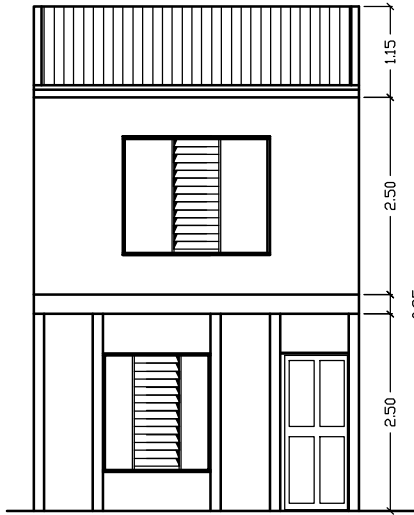
ELEVACION PRINCIPAL
